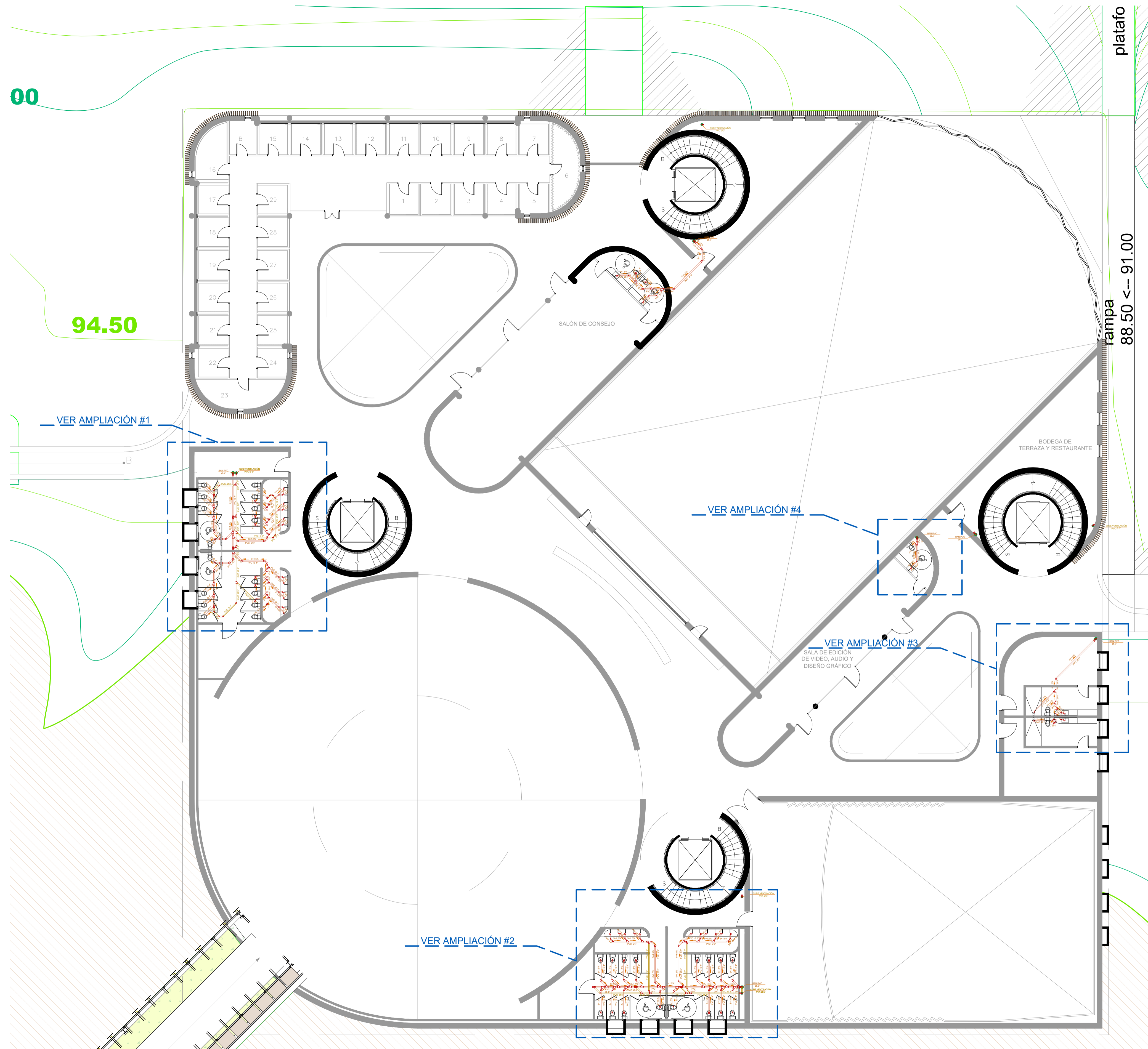
PLANO DE DRENAJES MEZZANINE -1 ESCALA 1 : 150
